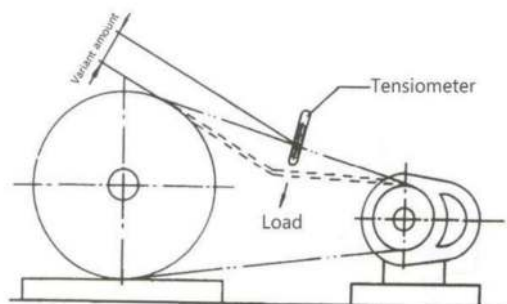
Подписи к рисунку: Колебания – Тензиометр – Нагрузка
